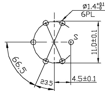
P.C.B LAYOUT(±0.1) (BOTTOM VIEW)
